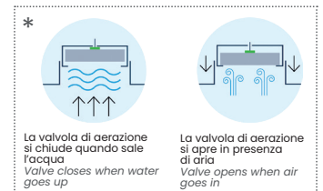
Valvolina di aerazione* Air ventilation valve*
